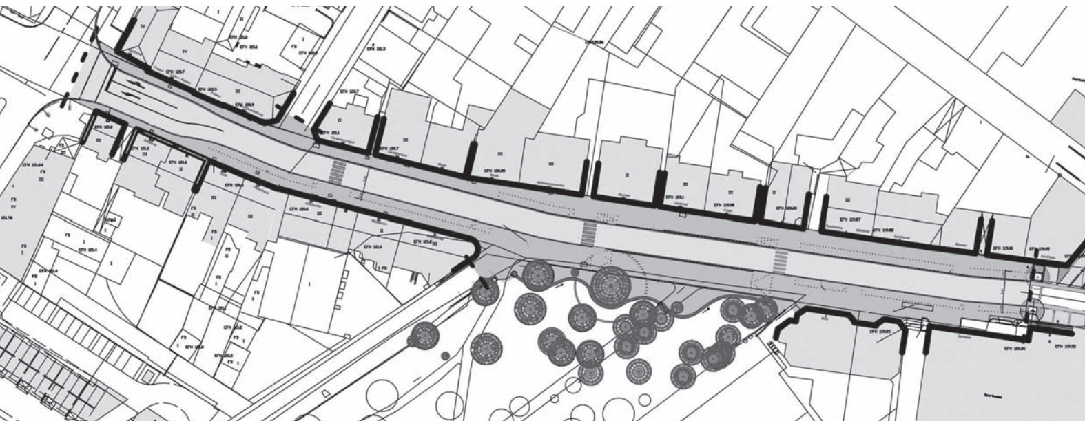
6.2.1 _Entwurf Bahnhofstraße
